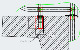
Variante A: Consola empotrada
