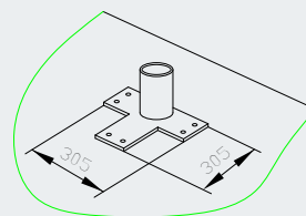
Variante B: Consola atornillada
